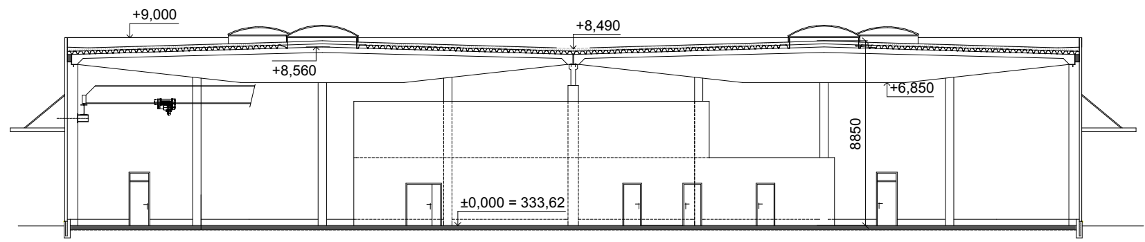
ŘEZ A - A - CUT A - A
